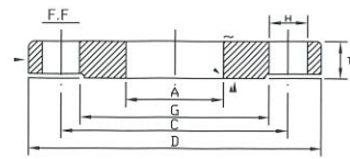
ANSI 125型 FLANGES
