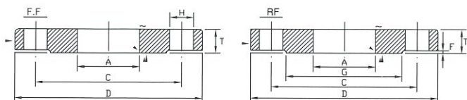
JIS 20kg/cm 2 型 FLANGES
