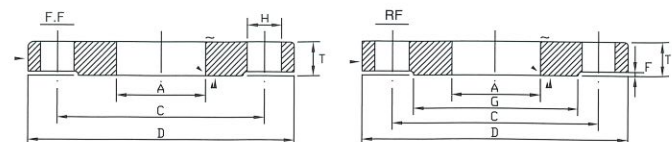
ANSI 300型 FLANGES
