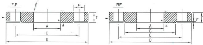
JIS 10kg/cm 2 型 FLANGES
